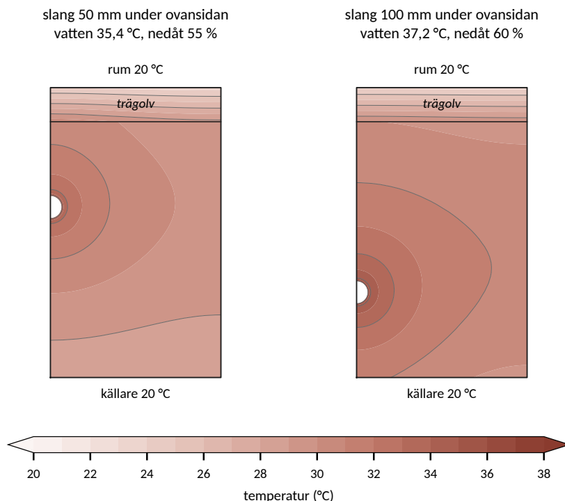
Figur 6: Temperatur i tvärsnittet med slangens högt (under överkantsnätet) och lågt (på underkantsnätet), källare 20 °C.
