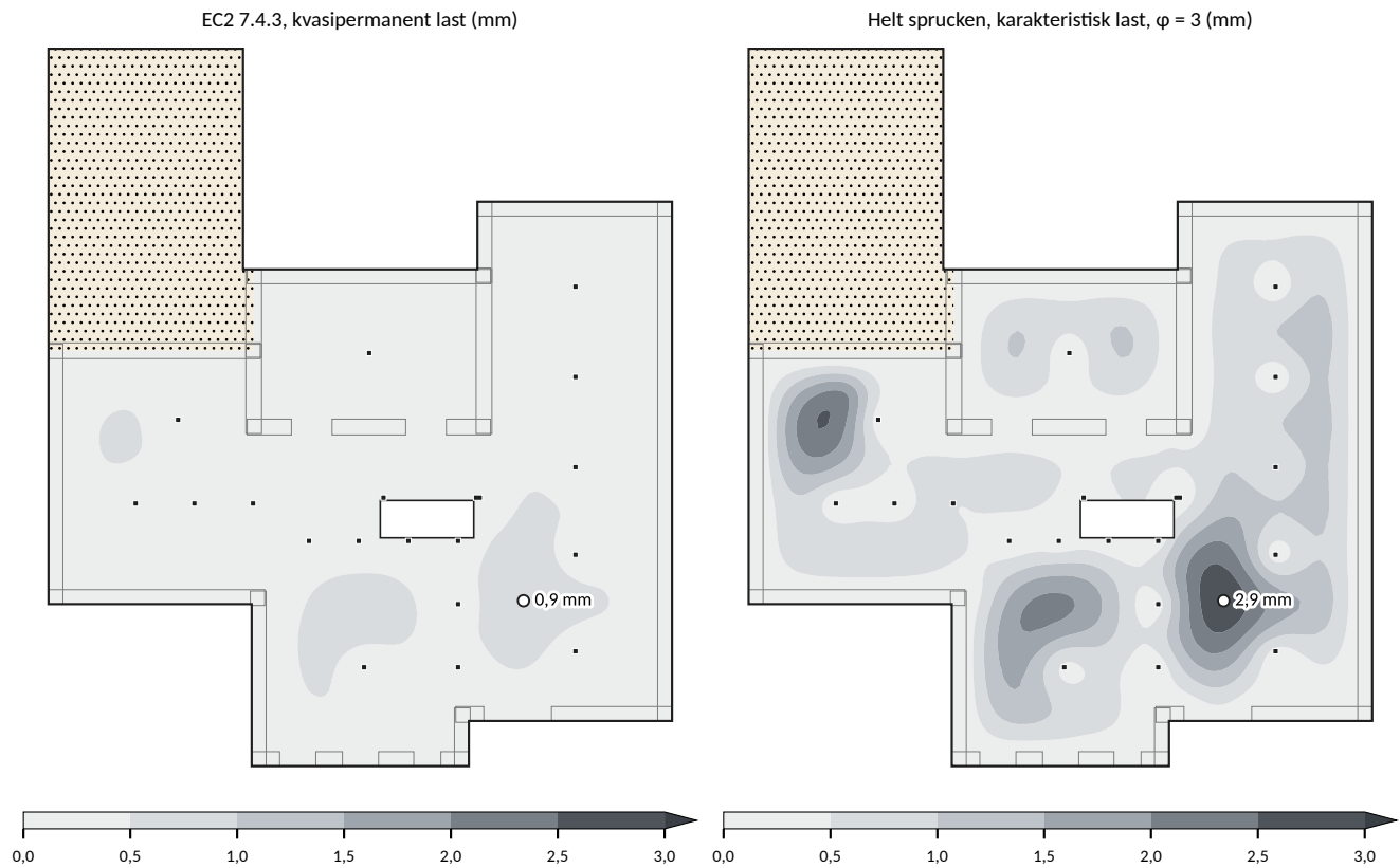
Figur 5: Långtidsnedböjning (mm). Rörens hoptryckning ingår.
