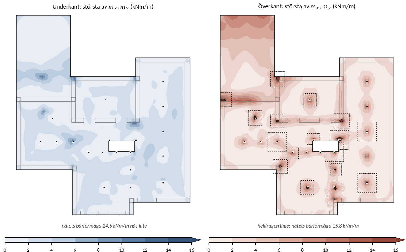
Figur 4: Dimensionerande moment i brottgränstillstånd, utjämnade över 250 mm (överkant \times 1,2 ), omhullande för alla kombinationer och de tre stödvarianterna (avsnitt 5). Heldragen linje: nätets bärförmåga. Streckat: zoner med tilläggsjärn.
