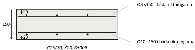
Figur 3: Plattans tvärsnitt, mm. Järnen i varje nät läggs i valfri ordning.
